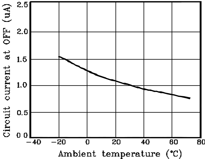
Fig. 6 I_{CCH} - T_a
